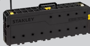
TAVOLO DA LAVORO RICHIUDIBILE ESSENTIAL WORKBENCH DIMENSIONI: APERTO: 80X61X73,6 CHIUSO: 85X30X16 CM ART.STST83492-1
