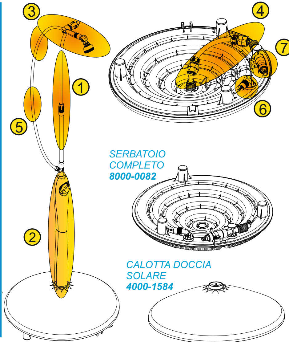
2_KIT COPRI MANOPOLA 4000-1940 BEIGE 4000-1943 VERDE
